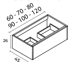
Soporte lavabo suspendido 1 cajón
