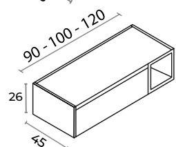
Bajo suspendido 1 cajón + 1 hueco decorativo (derecho o izq)
