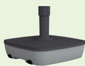
7767N11 25 L Base con ruedas. ø mástil 32-50 mm.
